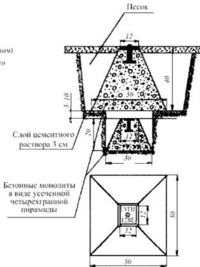
Соединение на цементном растворе
