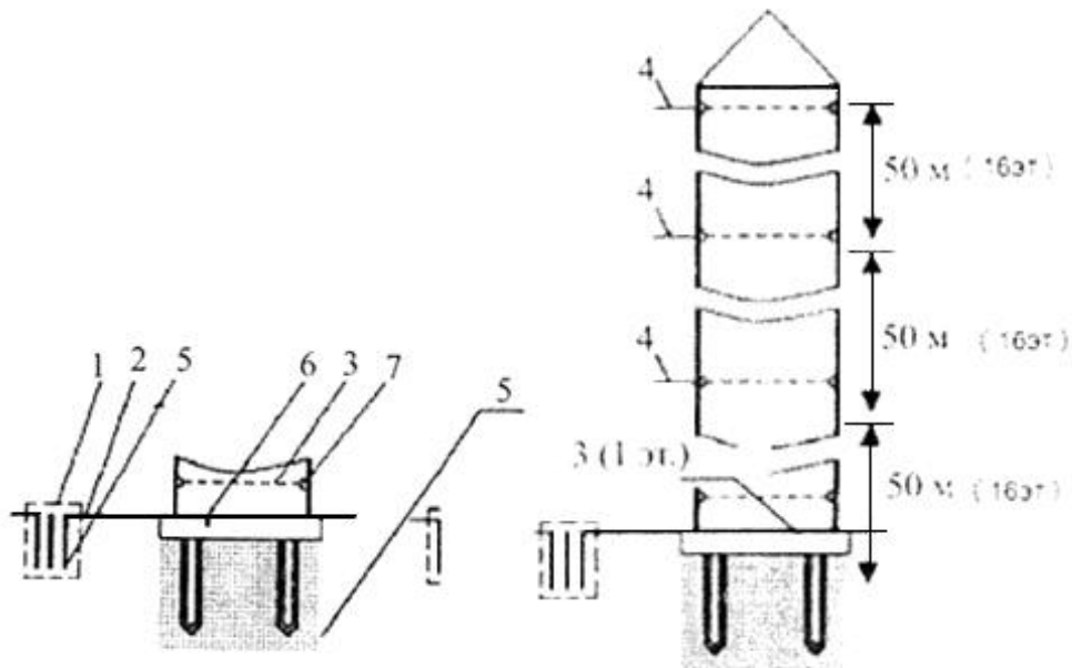
а) стадия возведения фундамента
