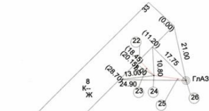
СХЕМА ПРИВЯЗОК Т.22-Т.26
