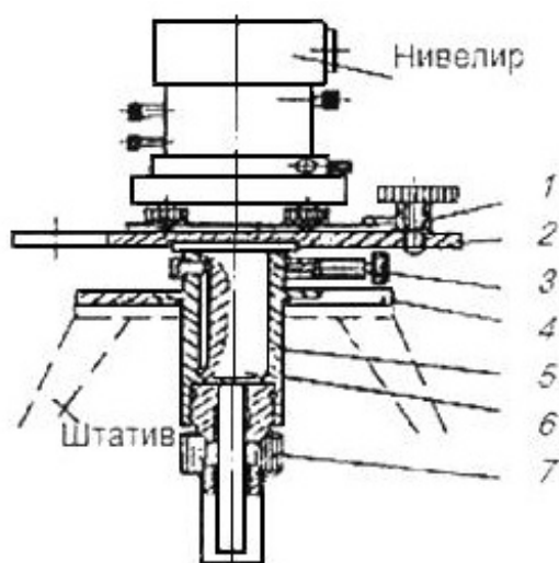
Рисунок И.1 - Прецизионная нивелирная подставка
